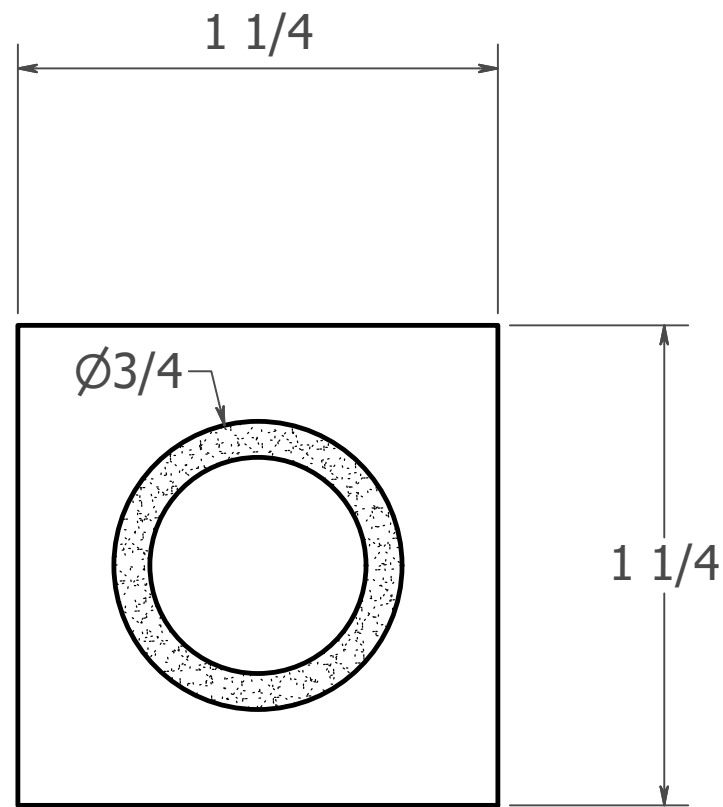
SECTION A-A SCALE 2 : 1
